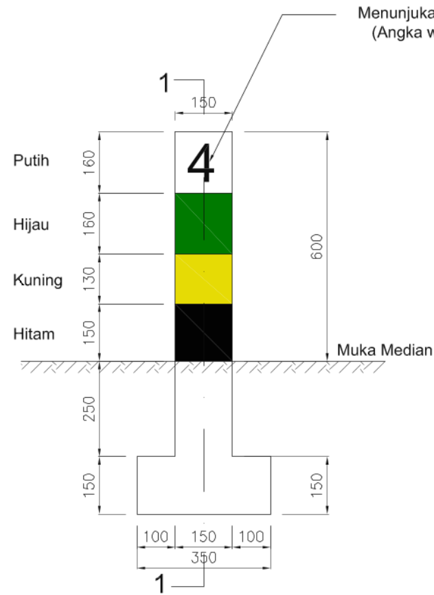
TAMPAK DEPAN
