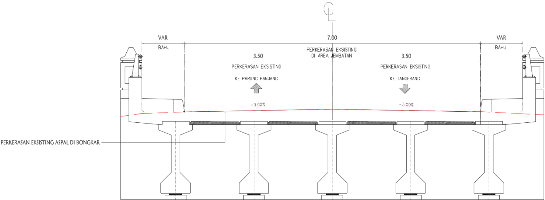
TIPIKAL POTONGAN EKSISTING SKALA 1:50
