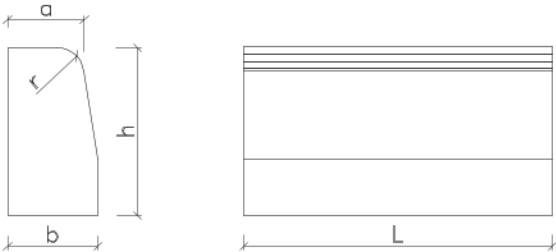
KEREB BIASA
