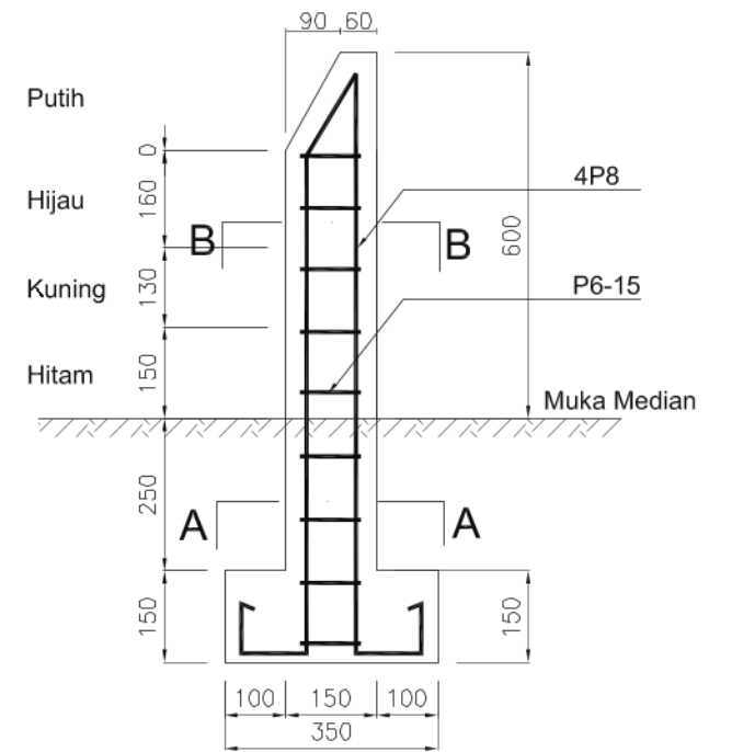
POTONGAN 1 - 1
