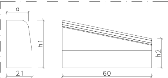
KEREB BIASA
