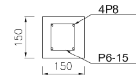
POTONGAN B - B
