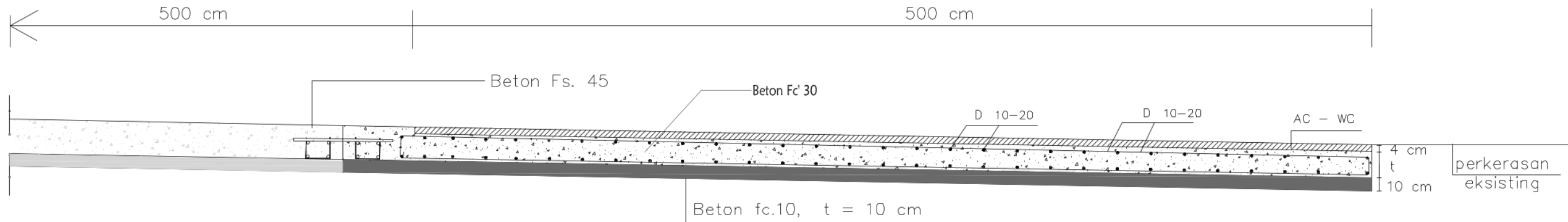
C. 6 DETAIL PERALIHAN PERKERASAN BETON KE PERKERASAN HOTMIX
