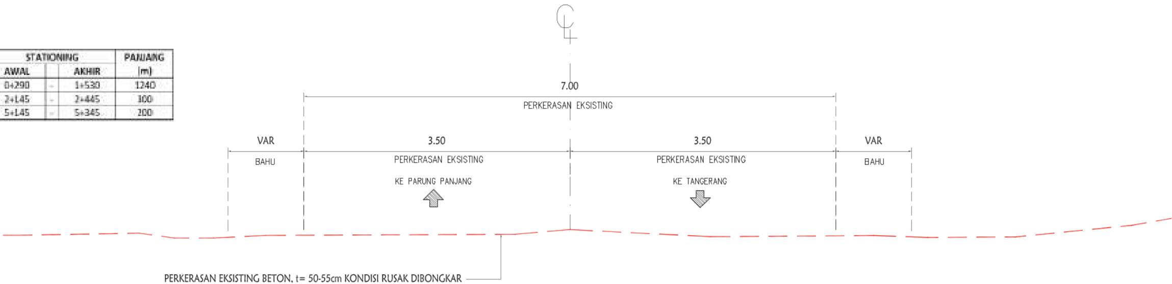
TIPIKAL POTONGAN EKSISTING SKALA 1: 50
