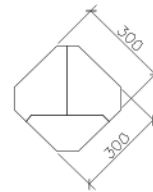
TAMPAK ATAS
