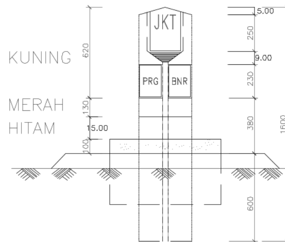
TAMPAK DEPAN
