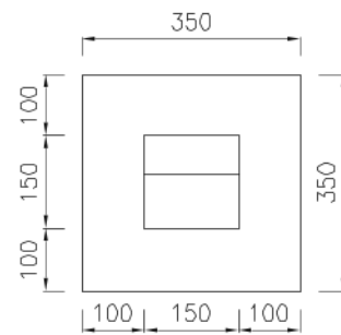
TAMPAK ATAS
