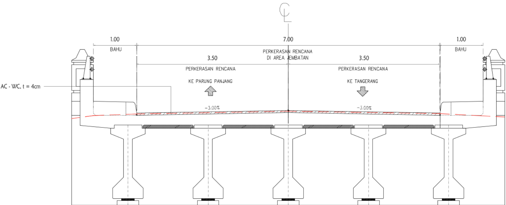
TIPIKAL POTONGAN RENCANA PERKERASAN ASPAL SKALA 1:50
