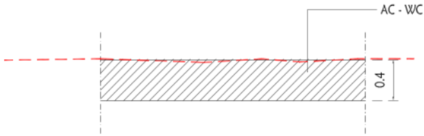
DETAIL PERKERASAN SKALA 1:25
