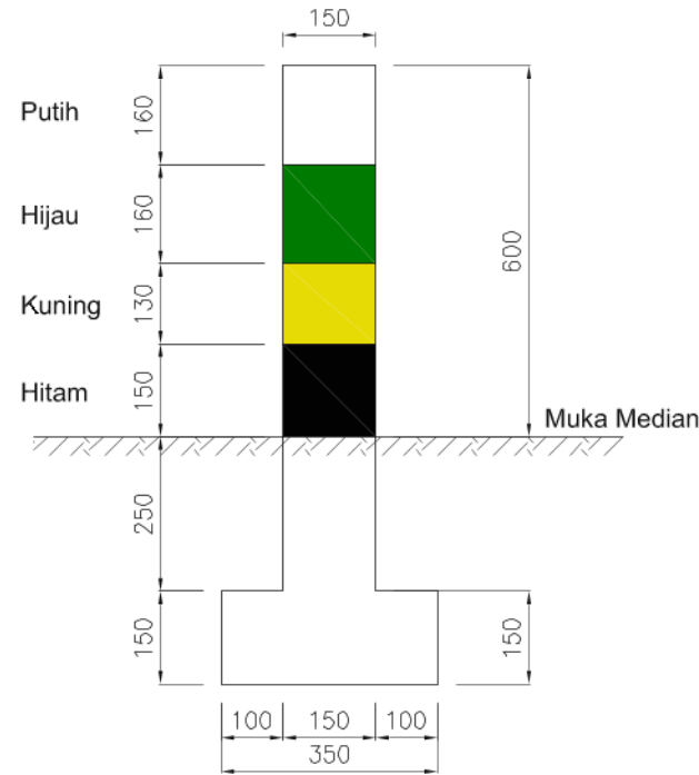
TAMPAK BELAKANG
