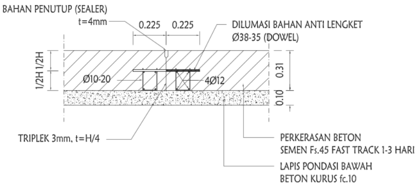
POTONGAN A SKALA 1: 25
